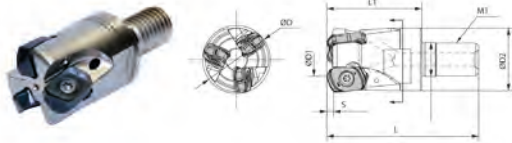
Raptor 04 Einschraubvariante
