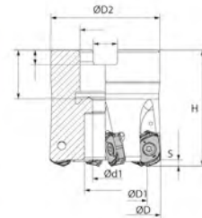
Raptor 04 Aufsteckvariante
